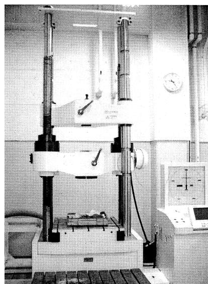
新しく導入した油圧サーボ 万能試験機
